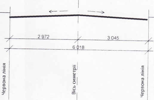
Поперечний профіль січення 1-1 М 1:100
